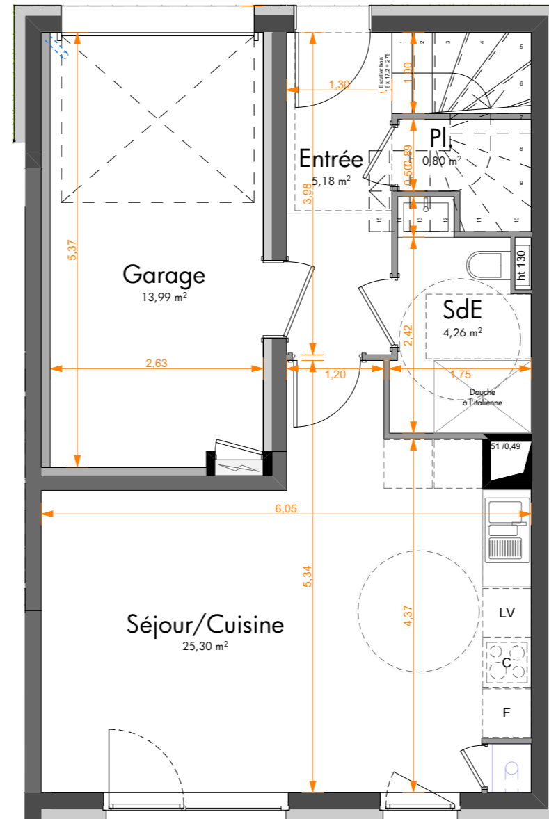
PLAN REZ-DE-CHAUSSEE
